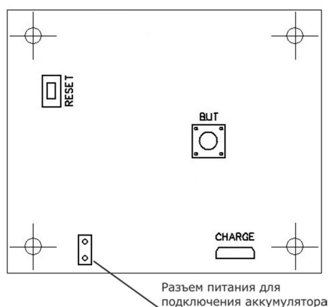
Рисунок 6.1. Внешний вид платы радиокнопки вызова MP-413W14
