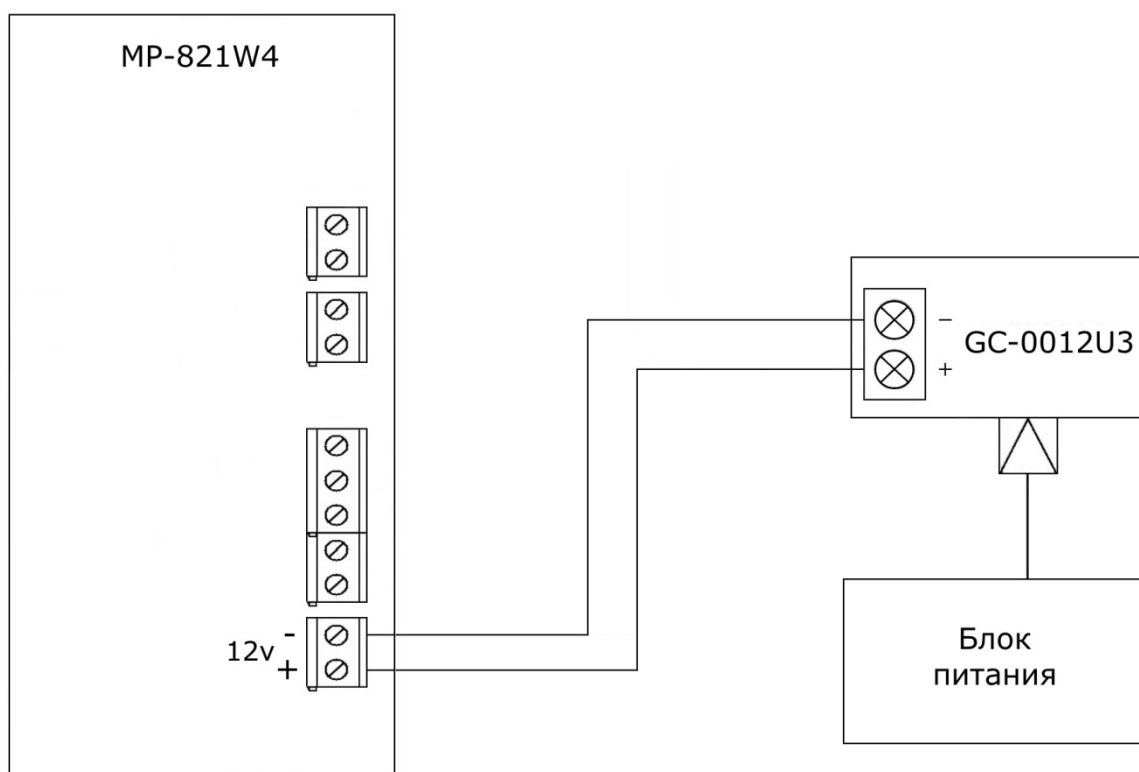
Рисунок 6.4. Схема соединений комплекта MP-920W14
